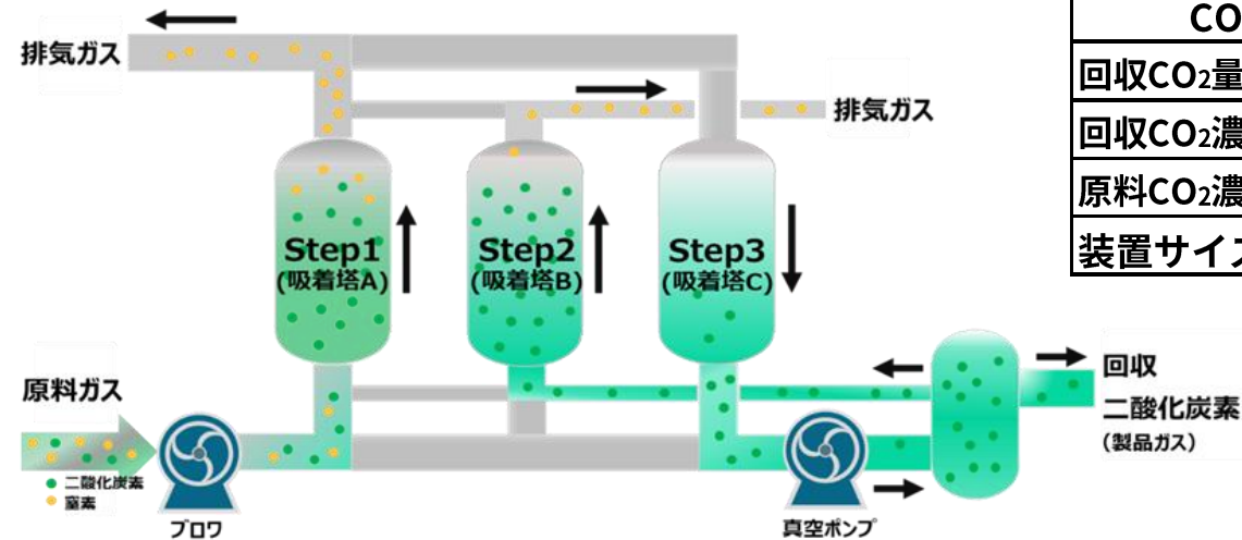
系統図
